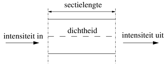
Figuur 1: De wet van behoud van voertuigen houdt in dat het aantal voertuigen dat in een bepaalde tijd een wegsectie oprijdt minus het aantal dat eraf rijdt gelijk is aan de toename van het aantal voertuigen op die sectie. De toename gedeeld door de lengte van de wegsectie is de toename van de dichtheid. De wet van behoud van voertuigen legt dus een verband tussen de macroscopische grootheden intensiteit en dichtheid .
